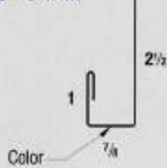
15 - J Trim
