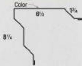
9 - Shadow Rake Trim
