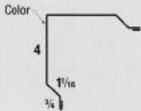
5 - Soffit
