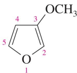
3-methoxyfuran
